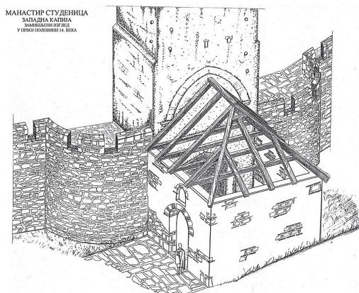
Сл. 6. Западна капија после доградње улазног анекса – замишљени изглед
