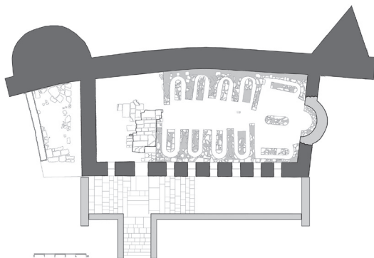
Сл. 2. Манастирска трпезарија – основа са етапама грађења
