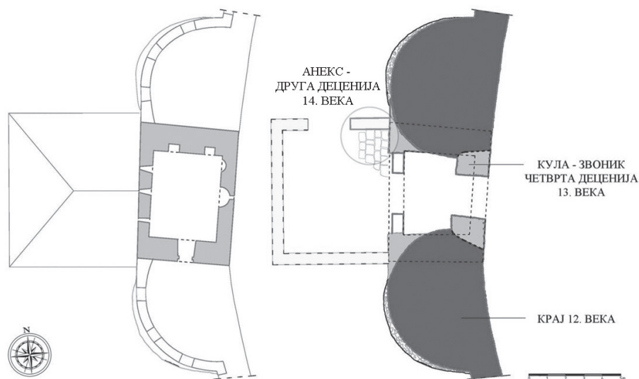
Сл. 5. Западна капија – основа са етапама грађења
