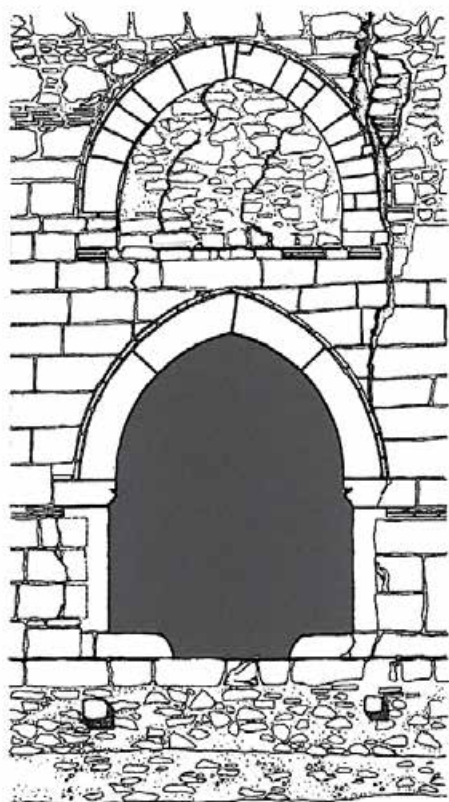
25. Главна кайија на Јужном бедему Смедеревског града – изглед и њресек (P=1:100)
