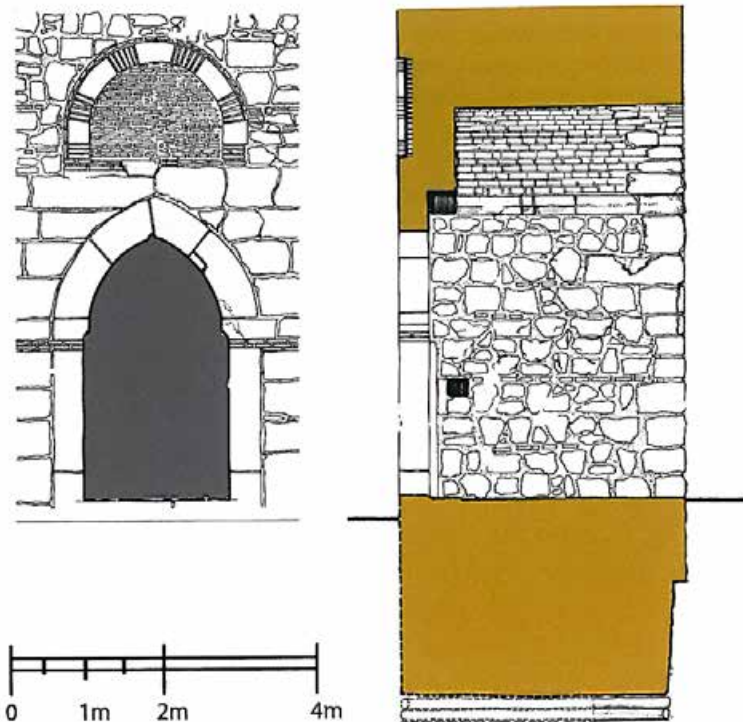
26. Језавска капија Смедеревског града – изглед и њресек ( P=1:100 )
