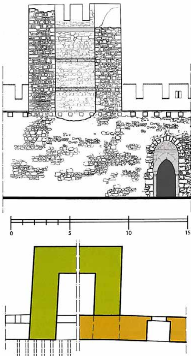
24. Кула 24 са кацијом на Дунавском бедуу Смедеревског града – основа и унутрашњи изглед ( P=1:200 )
