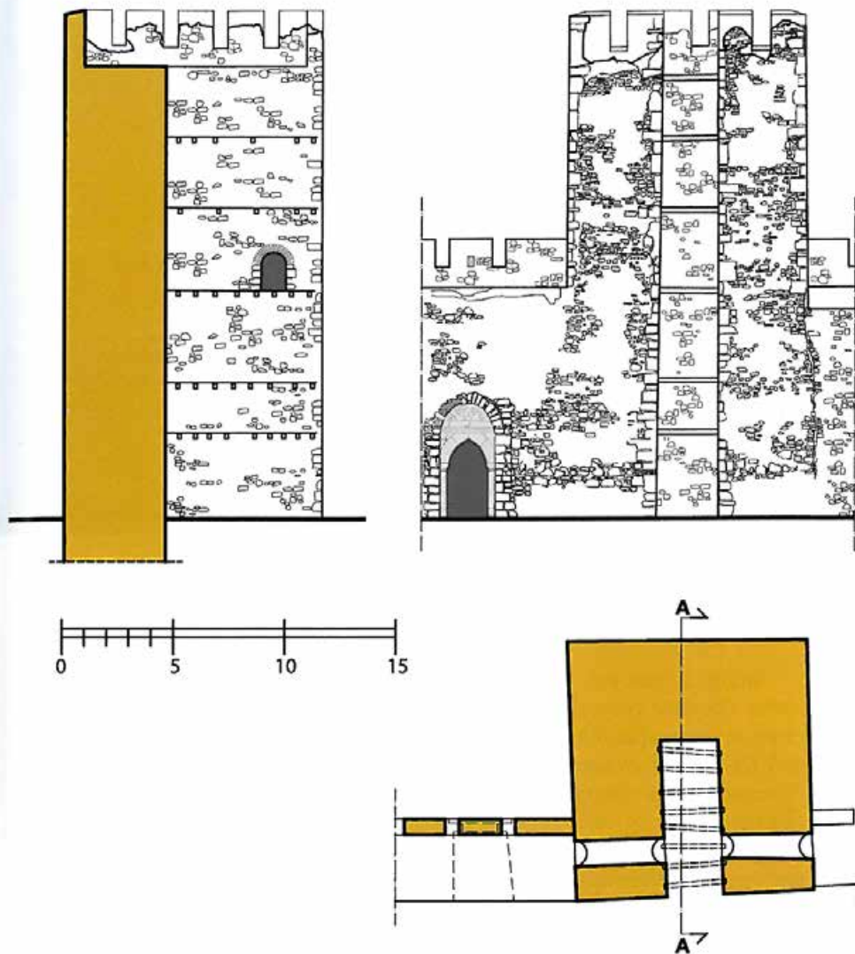
22. Кула 7 са кацијом на Језавском бреду Смедеревског града – основа унутрашњи изглед и пресек (P=1:300)
