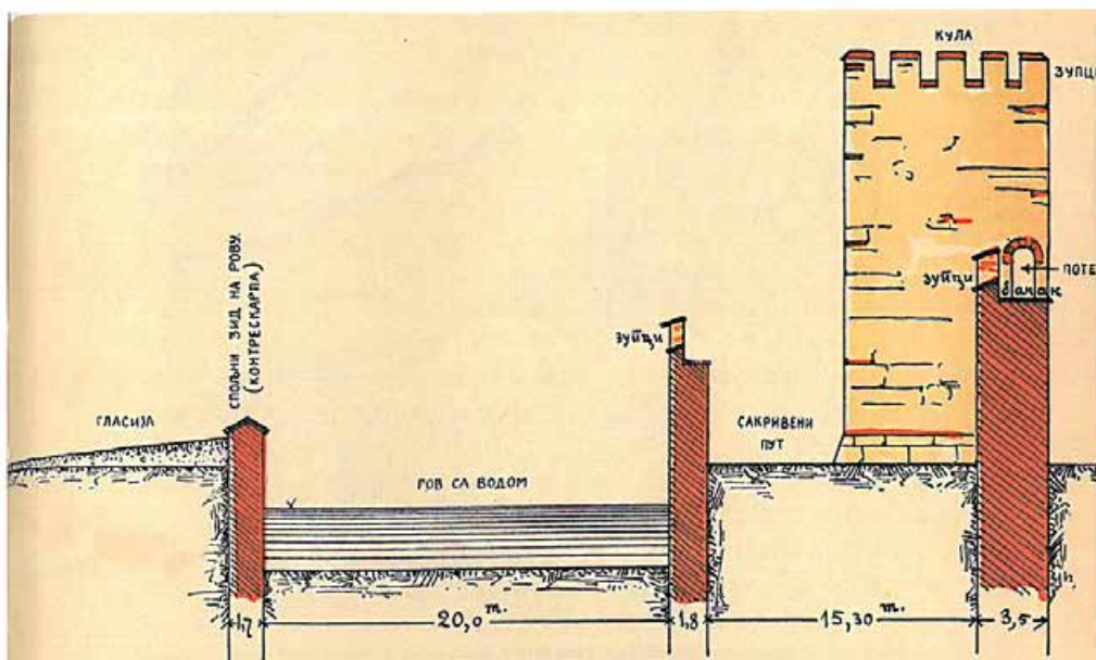
37. Јужни бедем Смедеревског града – пресек кроз систем фортификација
