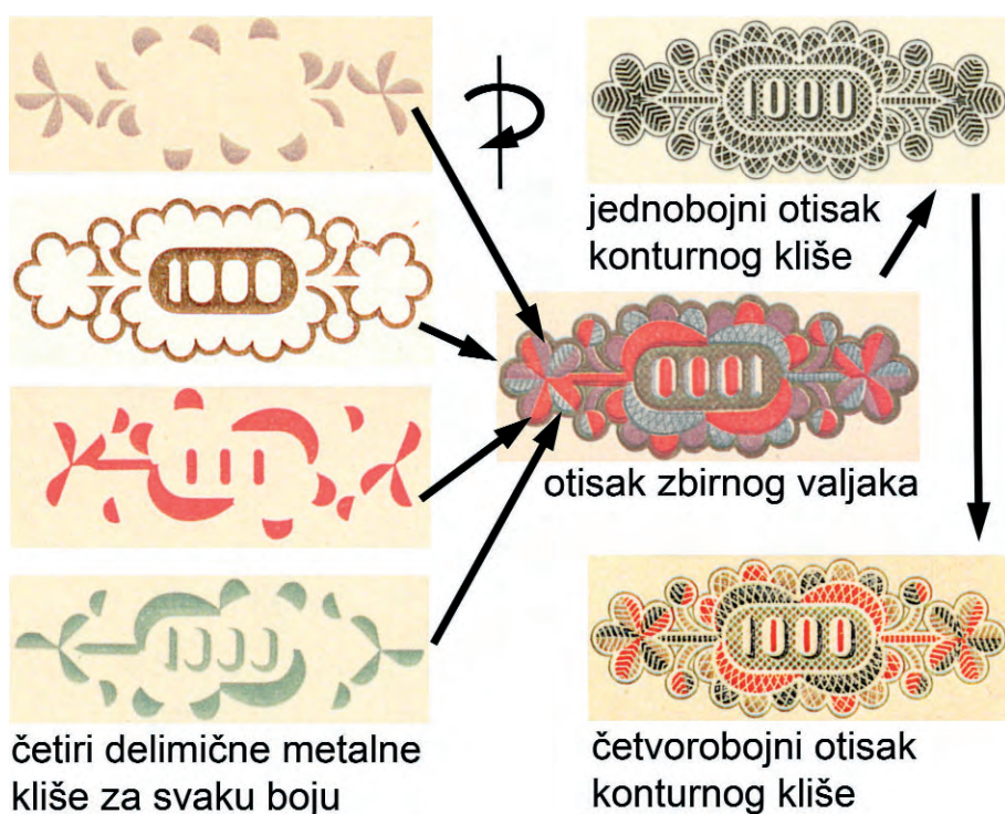
sl. 8. Šema prenosa boja iz delimičnih klišea na zbirni valjak i iz njega na hartiju pri orlovskoj štampi.
