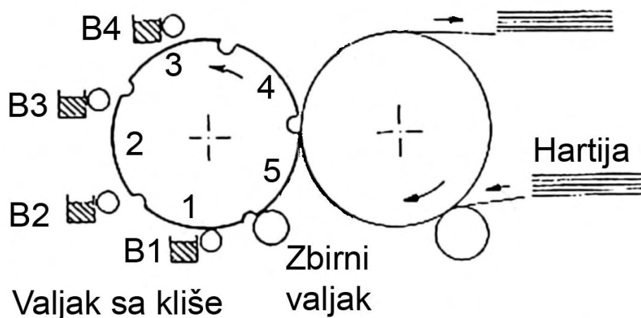
sl. 7. Uprošćena šema mašina za orlovsku štampu (B1 - B4), četvorbojni valjci za pojedinačne boje.
